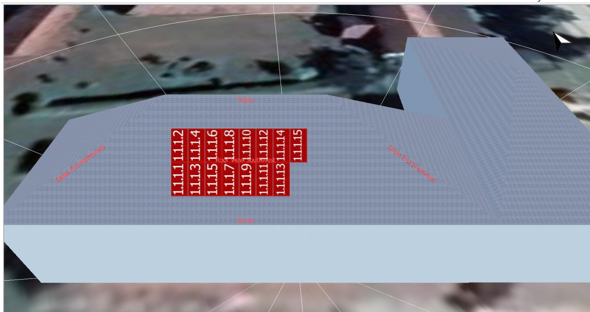
Slika 6: prikaz spajanja stringova
