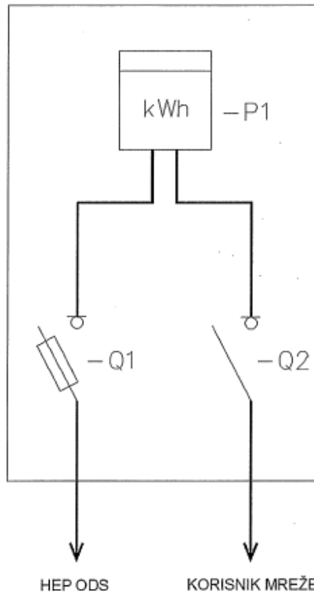
Slika 1. Priključno mjerni ormar (PMO) za 1 OMM, smjer proizvodnje: P \leq 50 kW, smjer potrošnje: P \leq 50 kW (izravno mjerenje) – za sunčane elektrane
