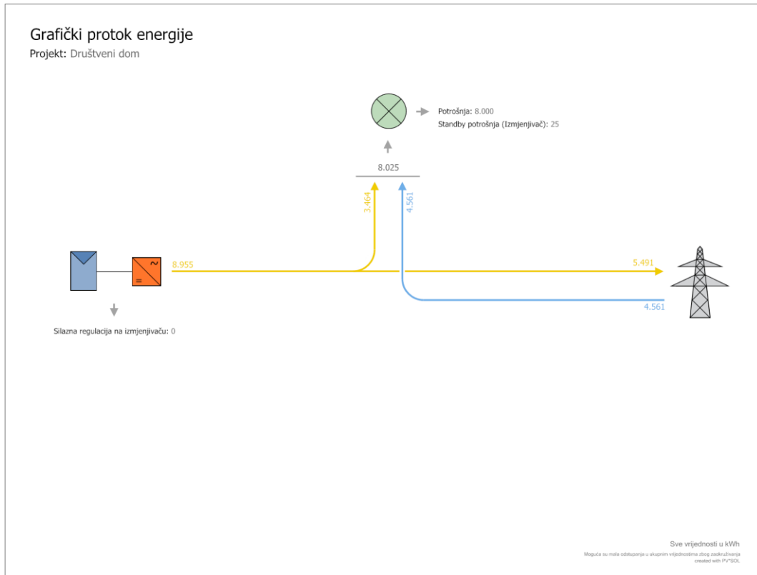
Slika 7: Protok energije
