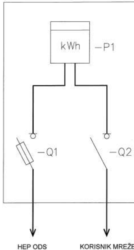
Slika 6. Priključno mjerni omar (PMO) za 1 OMM, smjer proizvodnje: P \leq 50 \text{ kW} , smjer potrošnje: P \leq 50 \text{ kW} (izravno mjerenje) – za sunčane elektrane
