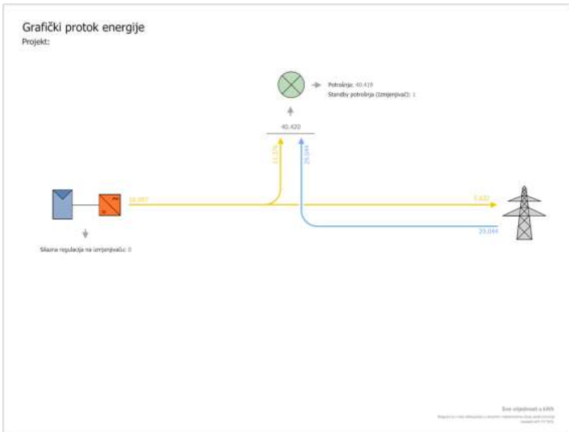
Slika 7: Protok energije
