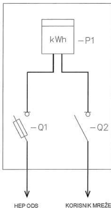
Slika 1. Priljučno mjerni omar (PMO) za 1 OMM, smjer proizvodnje: P \leq 50 \text{ kW} , smjer potrošnje: P \leq 50 \text{ kW} (izravno mjerenje) – za sunčane elektrane
